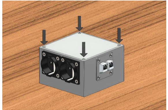
Schrauben lösen Deckel abnehmen
